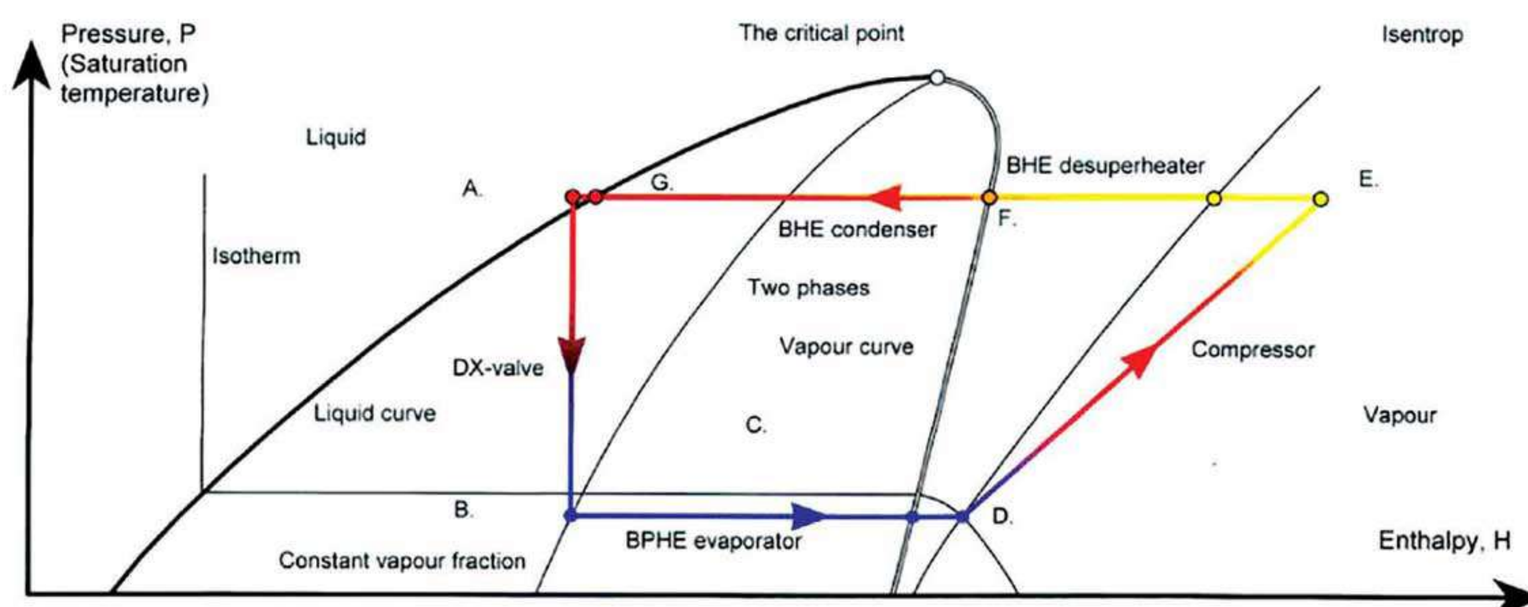
دیاگرام آنتالپی فشار سیکل تراکمی سرمایی
